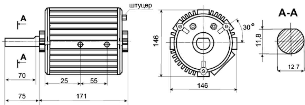
Рис. 1 исполнение АИРУ71А6.
