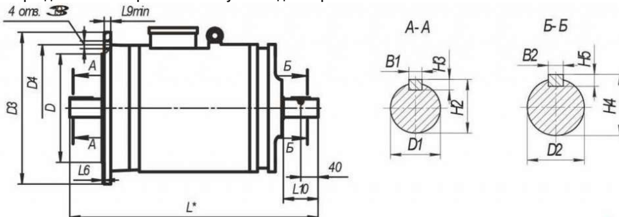
Размеры двигателей лифтовых малошумных односкоростных
